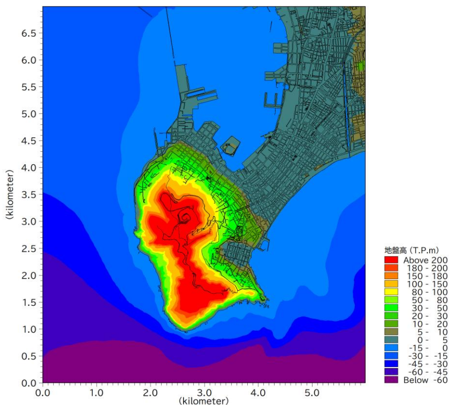
図- 8 10m 格子領域地形データの例(函館港周辺)
