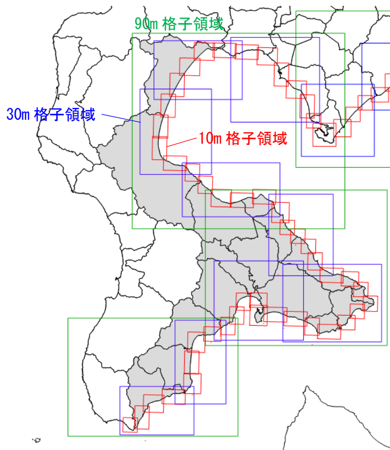
図-7 計算領域および計算格子間隔
