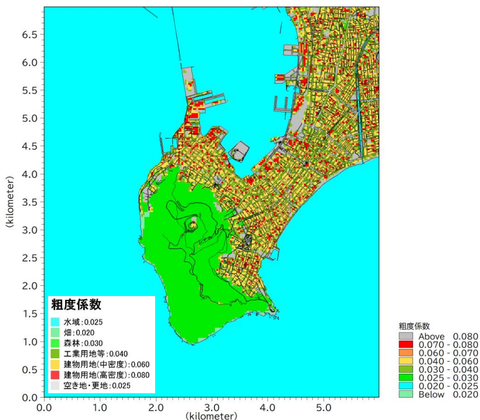
図-9 10m 格子領域粗度データの例(函館港周辺)
