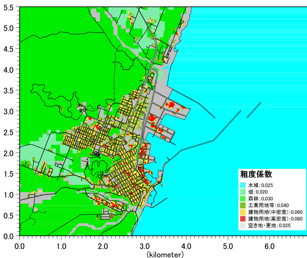
図- 9 10m 格子領域粗度データの例(十勝港周辺)
