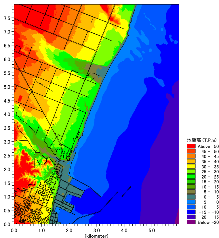
図- 8 10m 格子領域地形データの例(十勝港周辺)
