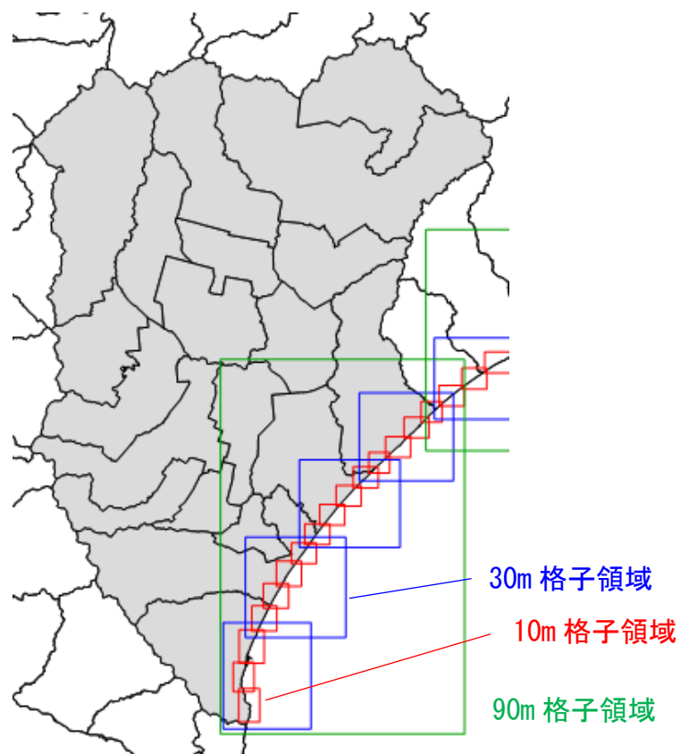
図-7 計算領域および計算格子間隔
