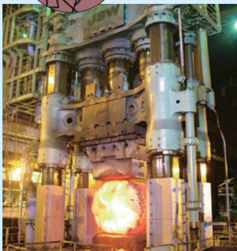
たんれん 鍛錬工場「1万4千トン水圧プレス」
